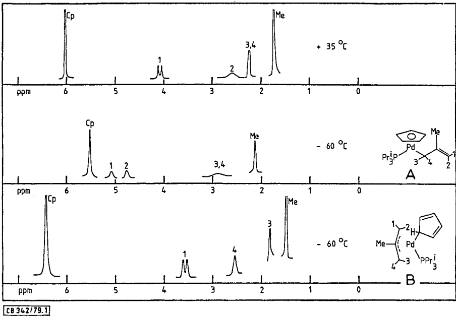
Abb. 1. 1 H-NMR-Signale der C 5 H 5 - und Allyl-Protonen von 4 bei 35 und -60 °C in [D 8 ]Toluol (die bei -60 °C beobachteten Signale der Isomeren A und B sind getrennt aufgeführt)
