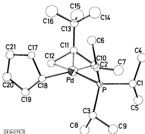
Abb. 3. Kristallstruktur von \text{C}_5\text{H}_5\text{Pd}(2\text{-t-BuC}_3\text{H}_4)\text{P}(\text{i-Pr})_3 (5)
