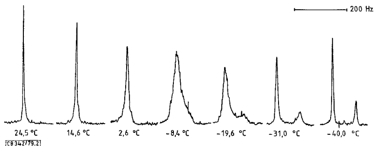
Abb. 2. Form des C_5H_5 -Signals von C_5H_5Pd(2-MeC_3H_4)PPhCy_2 ( 14 ) in [D_8]Toluol (100 MHz; die Signale im Koaleszenzbereich wurden mit erhöhter Verstärkung aufgenommen)
